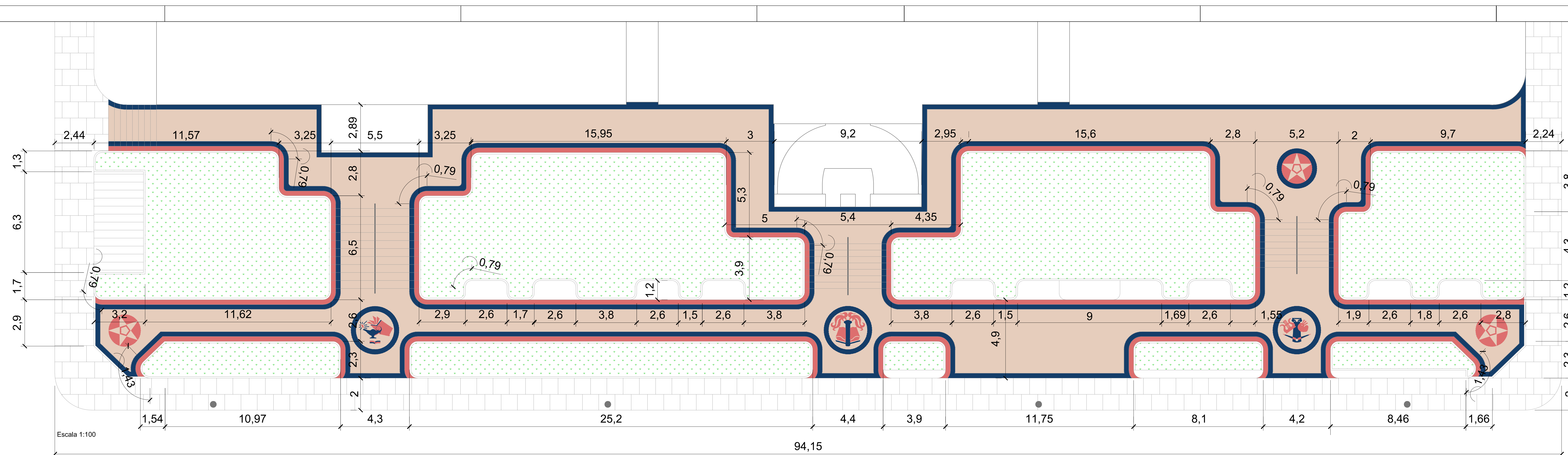
PLANTA BAIXA - IMPLANTAÇÃO - SITUAÇÃO ATUAL
